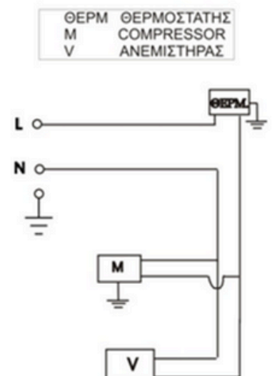
ΗΛΕΚΤΡΙΚΟ ΔΙΑΓΡΑΜΜΑ
